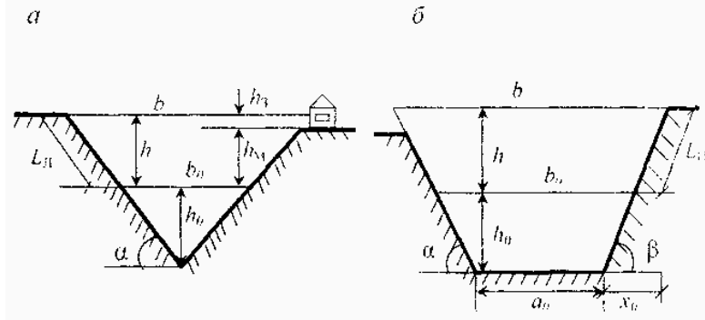
Рис. 3.1. Схема русла реки: a — треугольное русло; б -трапецидальное русло
