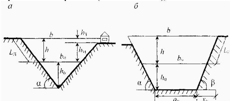
Рис. 3.1. Схема русла реки: а — треугольное русло; б — трапециевидное русло
