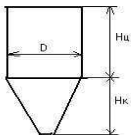
Рис.1. Расчетная схема бункера, состоящего из цилиндрической и конической частей
