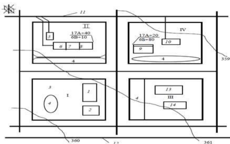
Рис. 2. Пример схемы генерального плана предприятия 1 – заводоуправление; 2 – столовая; 3 – стоянка автотранспорта; 4 – санитарно-защитная зона; 5 – депо; 6, 7, 8 – блок производственных цехов; 9, 10 – склады; 11 – железная дорога; 12 – автотдорога; 13 – ТЭЦ; 14 – АТС
