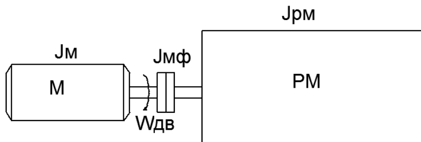
Рисунок 2. Кинематическая схема механизма
