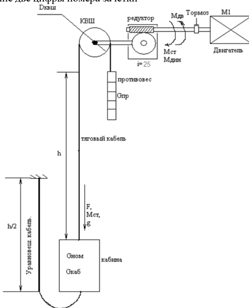
Рис 1. Кинематическая схема лифта
