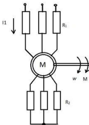
Рис. 1.3 Асинхронный двигатель с фазным ротором
