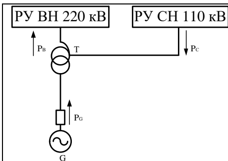
Рис. 1. Схема подключения автотрансформатора связи в блоке с генератором
