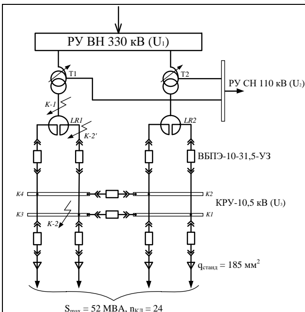
Рис. 1. Структурная схема подстанции 330/110/10 кВ с токоограничивающими реакторами
