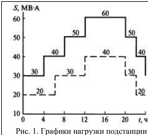
Рис. 1. Графики нагрузки подстанции
