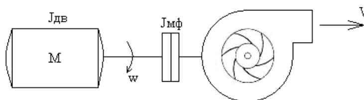
Рисунок 1.1 – Кинематическая схема центробежного насоса
