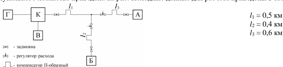
Рис. Схема теплоснабжения предприятий и объектов жилищно-коммунального хозяйства
