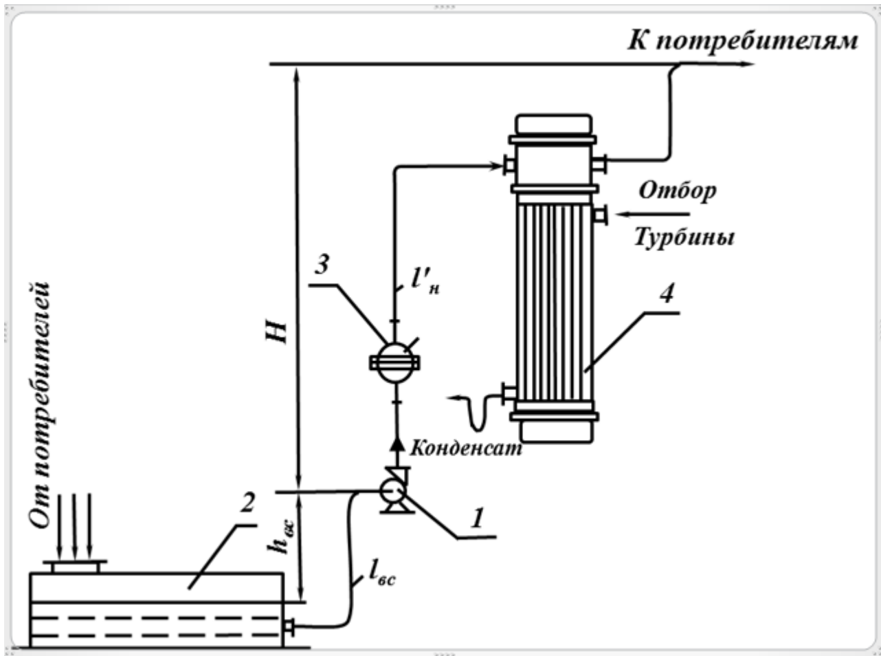
Рис.1 Теплотехнологическая схема
