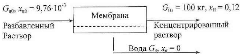
Схема процесса мембранного разделения
