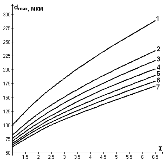
Рис.6. Зависимость величины d_{\max} при H = 0,4 м и L=0,25 м от коэффициента формы и плотности пылевых частиц
