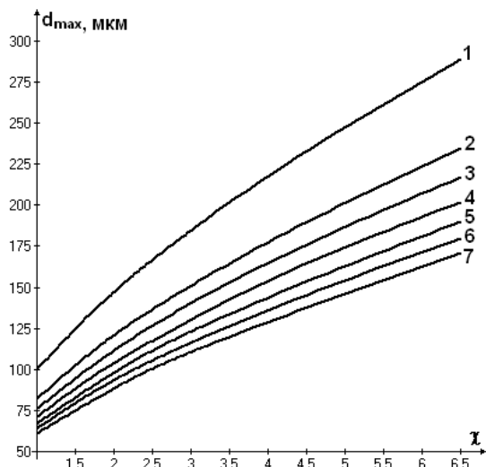
Рис.6. Зависимость величины d_{\max} при H = 0,4\text{м} и L=0,25\text{м} от коэффициента формы и плотности пылевых частиц
