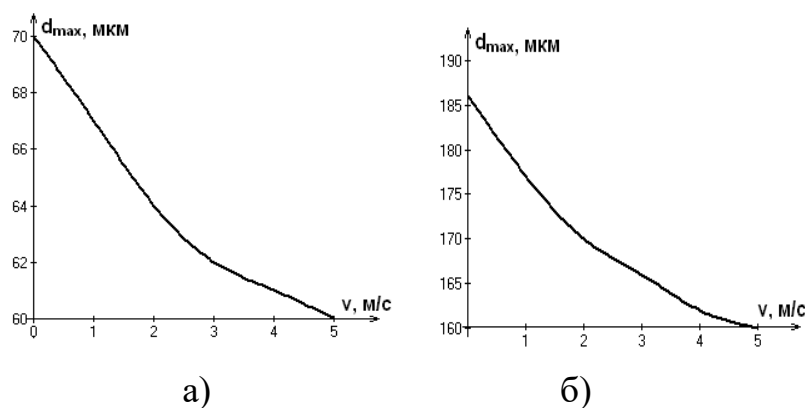
Рис.2. Зависимость величины максимального диаметра пылевой частицы от начальной скорости ее вылета: а – при \chi = 1 ; б – при \chi = 6
