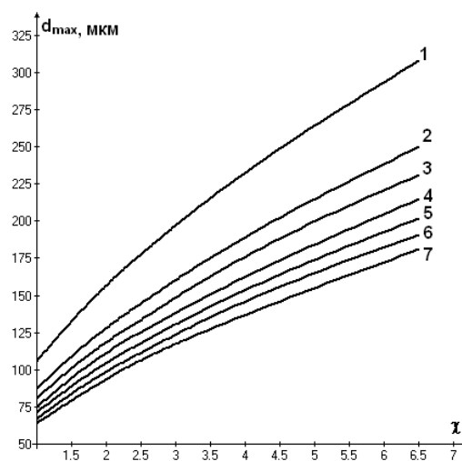
Рис.3. Зависимость величины максимального диаметра пылевой частицы от коэффициента ее формы и плотности: 1 – 1400 \text{ кг/м}^3 , 2 – 2000 \text{ кг/м}^3 , 3 – 2300 \text{ кг/м}^3 , 4 – 2600 \text{ кг/м}^3 , 5 – 2900 \text{ кг/м}^3 , 6 – 3200 \text{ кг/м}^3 , 7 – 3500 \text{ кг/м}^3
