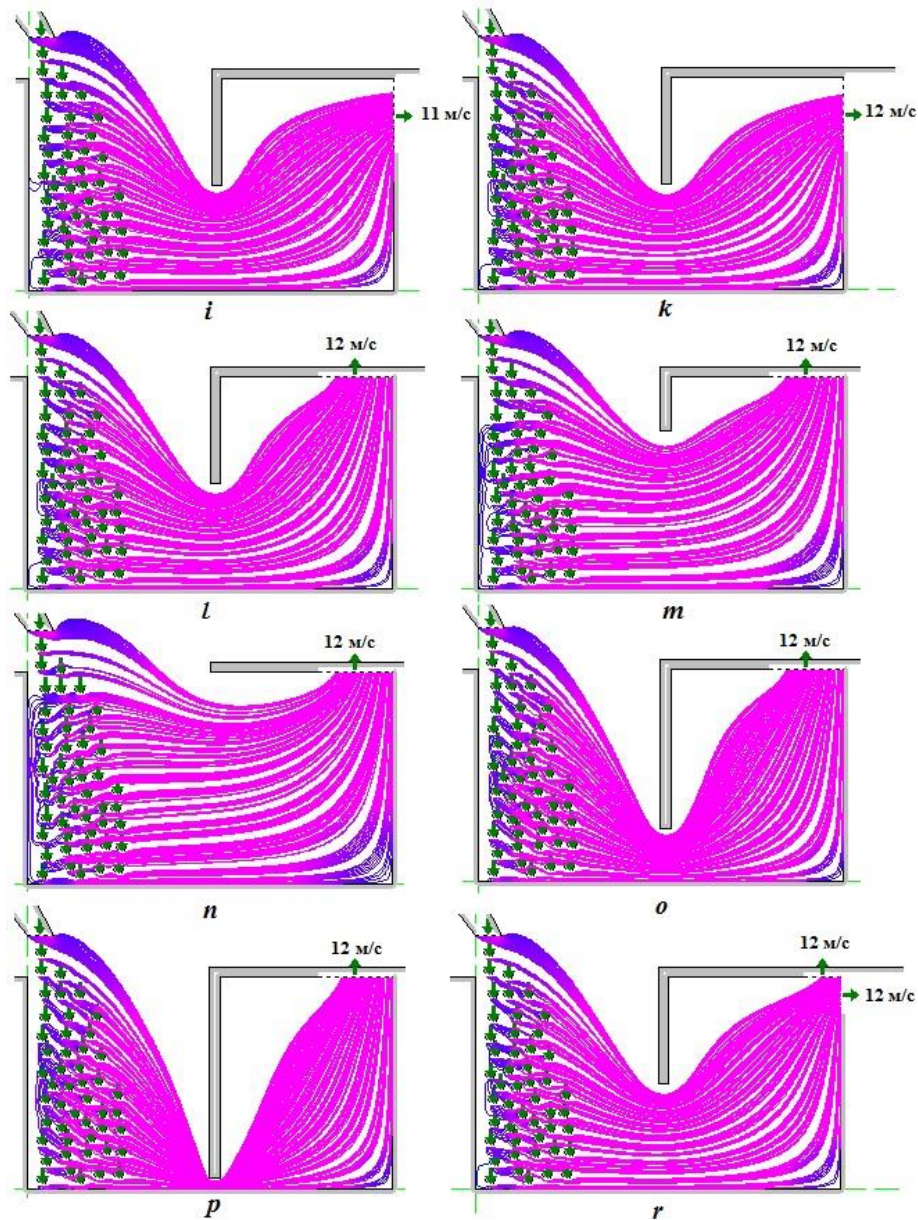
Рис.4. Линии тока: i ) m=0,1725\text{м}; l=0,1\text{м} ; k ) m=0,1725\text{м}; l=0,1\text{м} ; l ) m=0,1725\text{м}; l=0,1\text{м} ; m ) m=0,1725\text{м}; l=0,05\text{м} ; n ) m=0,1725\text{м}; l=0\text{м} ; o ) m=0,1725\text{м}; l=0,15\text{м} ; p ) m=0,1725\text{м}; l=0,15\text{м} ; r ) m=0,1725; l=0,15\text{м}
