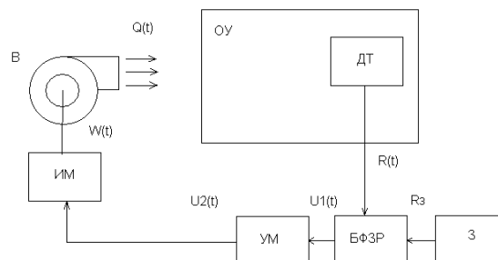
Рис.1 Функциональная схема системы автоматизации
