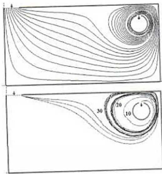
Рис.3. Линии тока и траектории пылевых частиц без цилиндра
