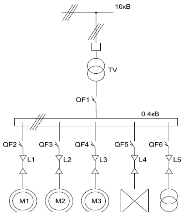
Рис. 1. Расчетная схема электроснабжения производственного объекта Примерные значения нагрузок подстанции представлены в табл. 1.
